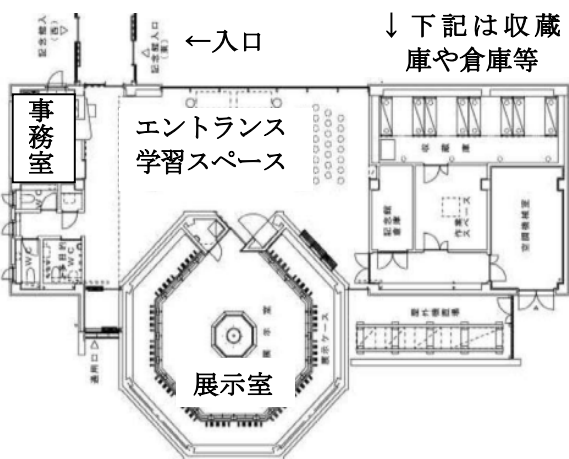
新塙記念館設計図 (上から見た配置)
